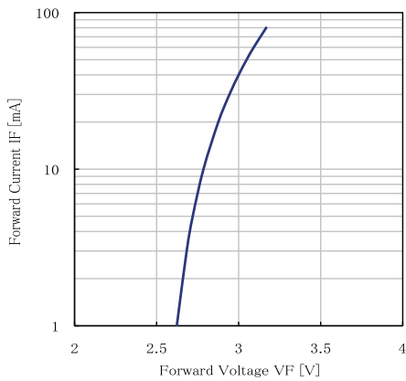
< I_F - V_F 特性 >
