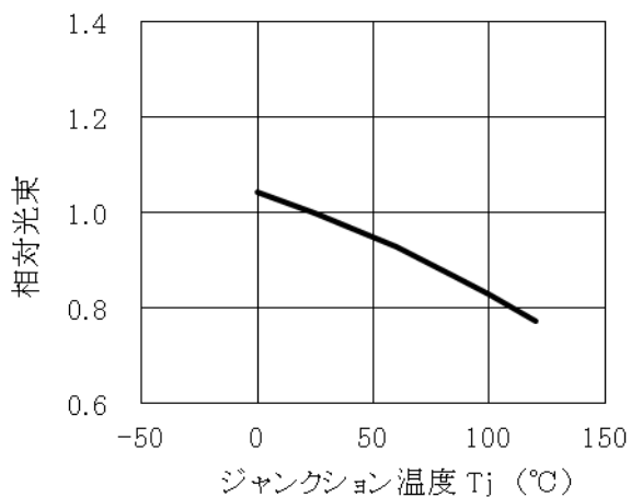
相対光束 - T_j ( I_F=65\text{mA} )
