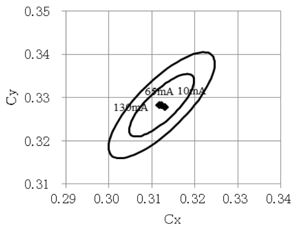
色度 - I_F ( T_a=25^\circ\text{C} )
